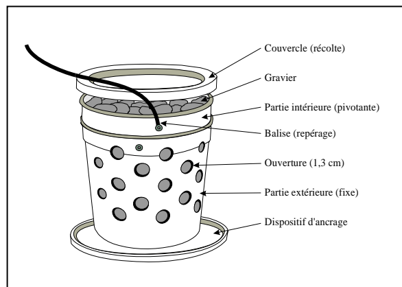
Figure 2 Collecteur de sédiments Sédibac
